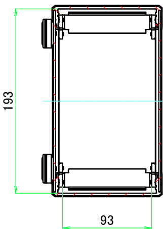
B-B ( 1 : 4 )
