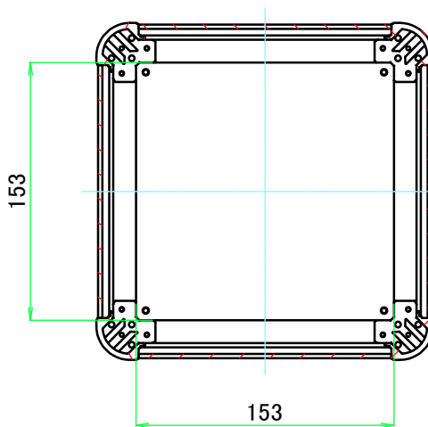
C-C ( 1 : 4 )
